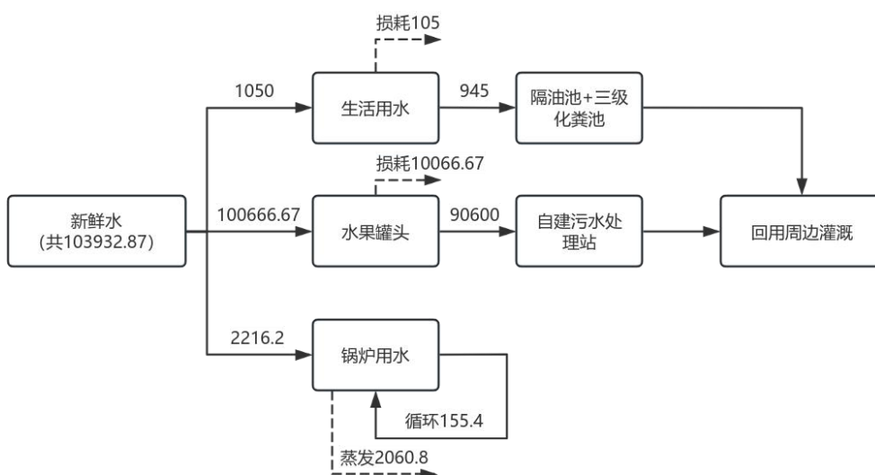
图 2-2 项目远期水平衡图 (t/a)
