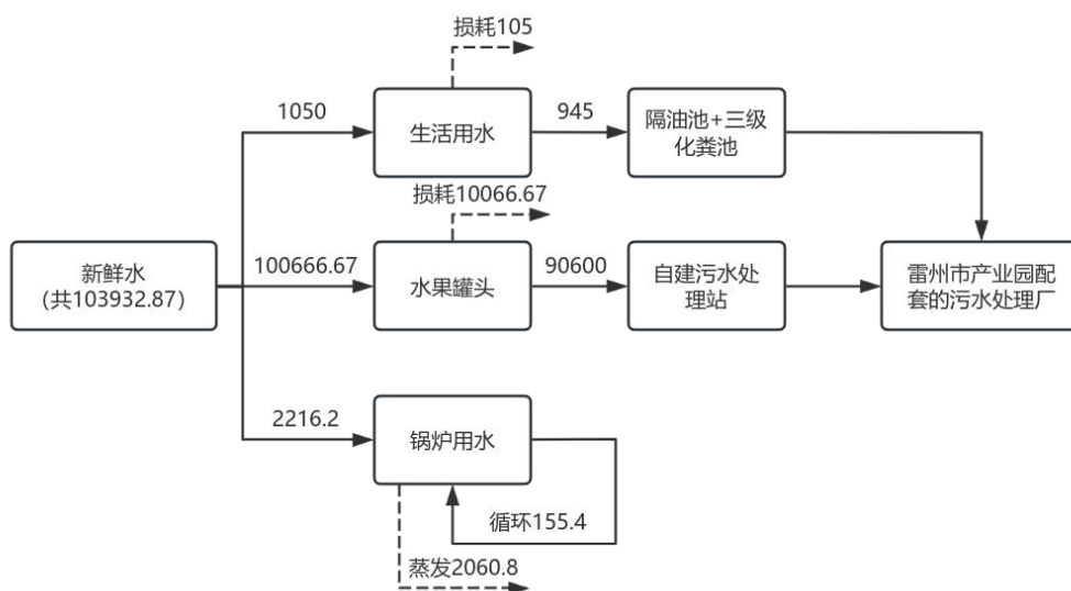
图 2-1 项目远期水平衡图 (t/a)
